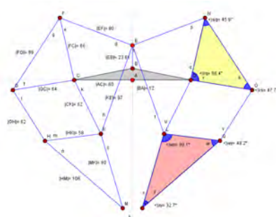
Figura 1 – Mecanismo de Jansen no Geogebra
