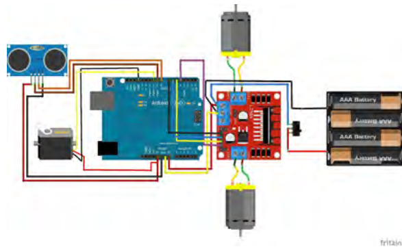
Figura 1 – Esquema do carro inteligente com as conexões (parte física)
