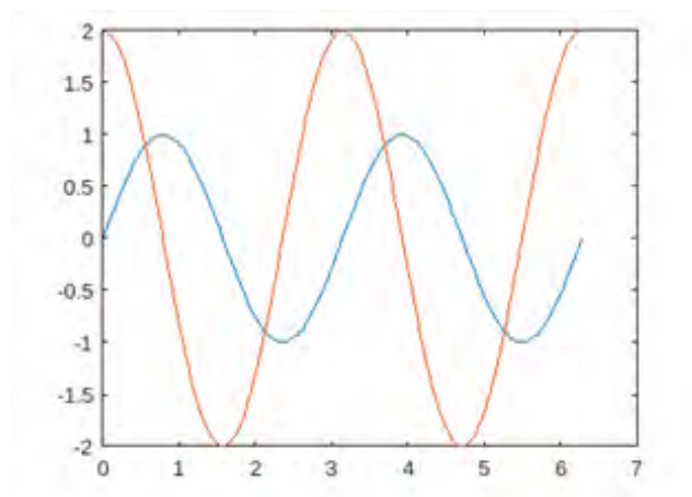
Gráfico 1 – Diagrama de f(x) = \sin(2x) e f(x) = 2 \cos(2x) .
