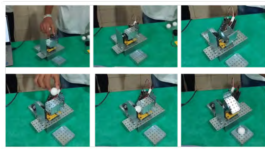
Figura 8 – Sequência de imagens extraída dos vídeos da demonstração do funcionamento do Separador de Lixo Automático.
