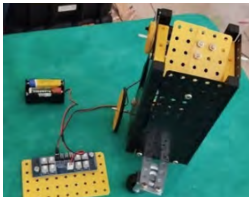
Figura 2 – Lixeira Automatizada construída pelos estudantes.
