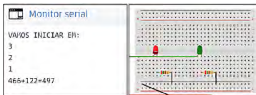
Figura 1 – Igualdade apresentada no monitor serial e resposta da igualdade com sinal luminoso de LED
