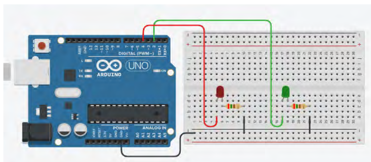
Figura 2 – Montagem do circuito no simulador Tinkercad .
